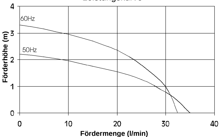
Leistungskurve*
